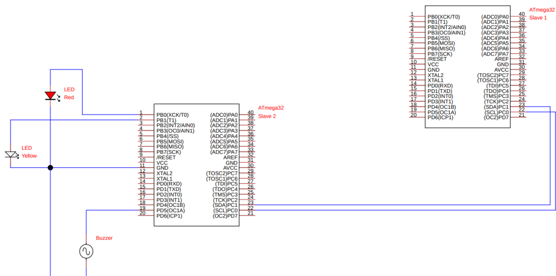
Figur 3: Digitalt koblingsskema – Slave 2 (reaksjon)
